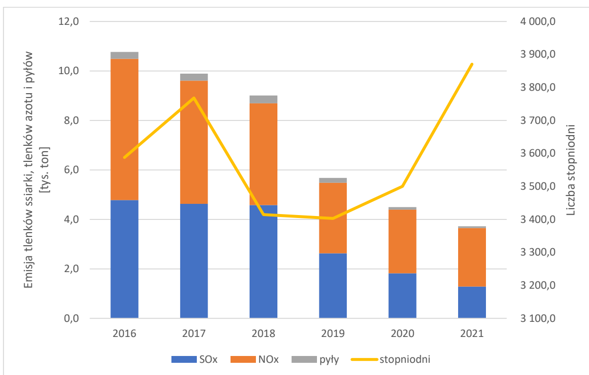
Rysunek 62 Emisja tlenków azotu (NOx), tlenków siarki (SOx) oraz całkowitych pyłów zawieszonych (TSP) na terenie miasta Kraków w latach 2016-2021 zaraportowane przez wytwórców energii.
