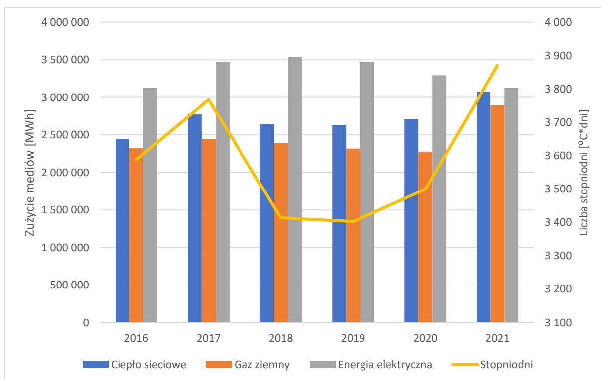
Rysunek 55 Zużycie nośników energii na terenie Krakowa w latach 2016-2021.
