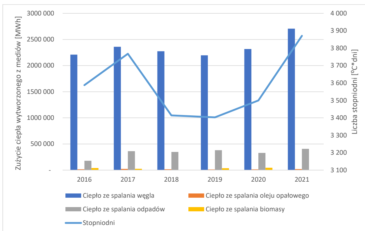
Rysunek 56 Zużycie energii cieplnej z poszczególnych paliw w latach 2016-2021.
