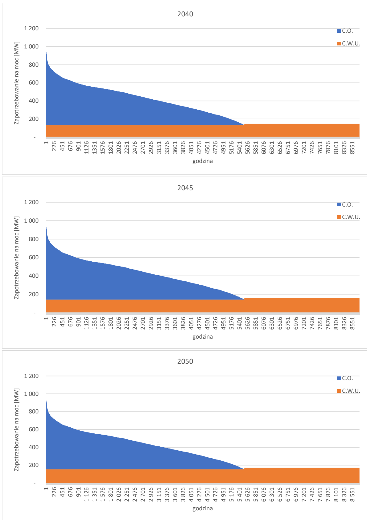
Rysunek 88 Porównanie wykresów uporządkowanych zapotrzebowania na produkcję ciepła w wybranych latach w okresie 2023 - 2050 w podziale na c.o. i c.w.u. według Scenariusza 1 bazowego. Źródło: Opracowanie własne KAPE S.A.
