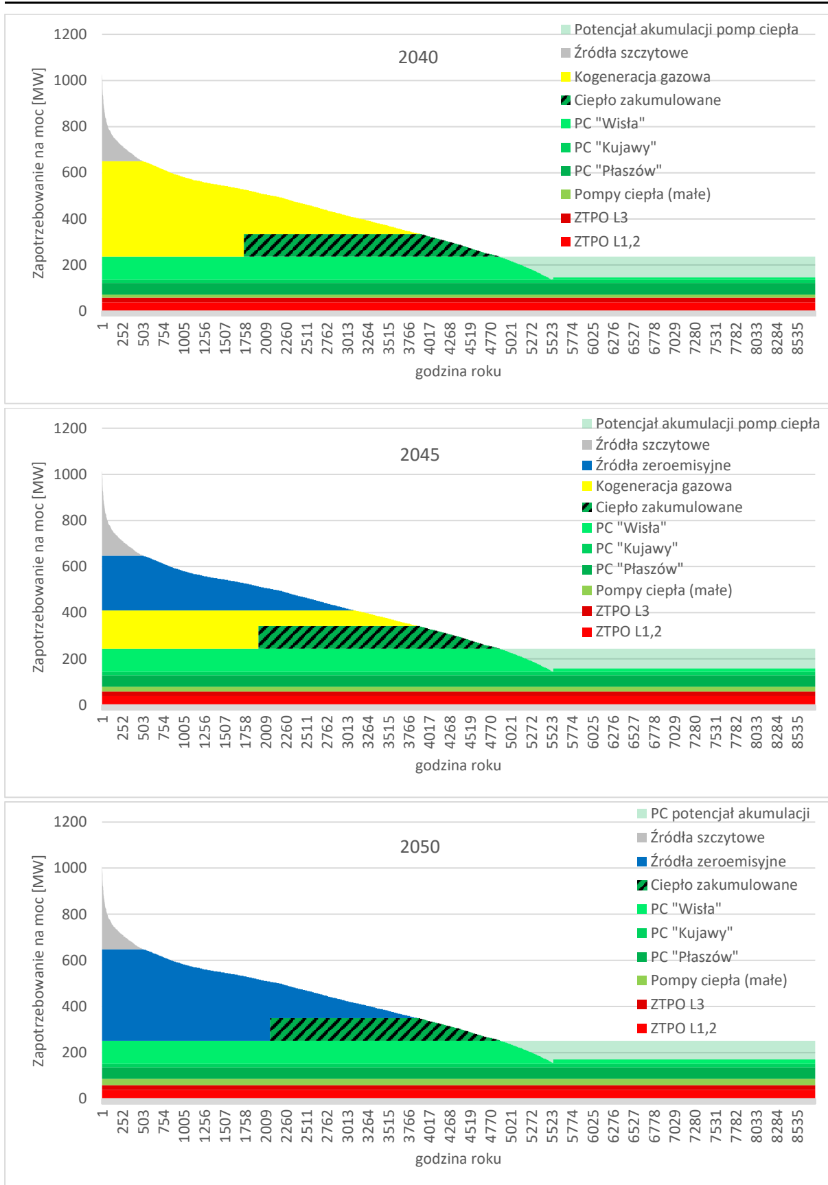
Rysunek 90 Porównanie wykresów uporządkowanych produkcji ciepła dla systemu ciepłowniczego w wybranych latach w okresie 2023 – 2050 według Wariantu.
