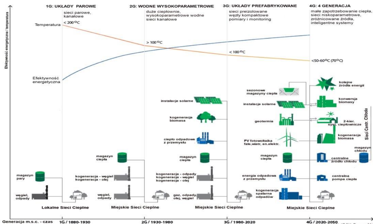
Rysunek 87 Prognozowane etapy rozwoju ciepłownictwa.
