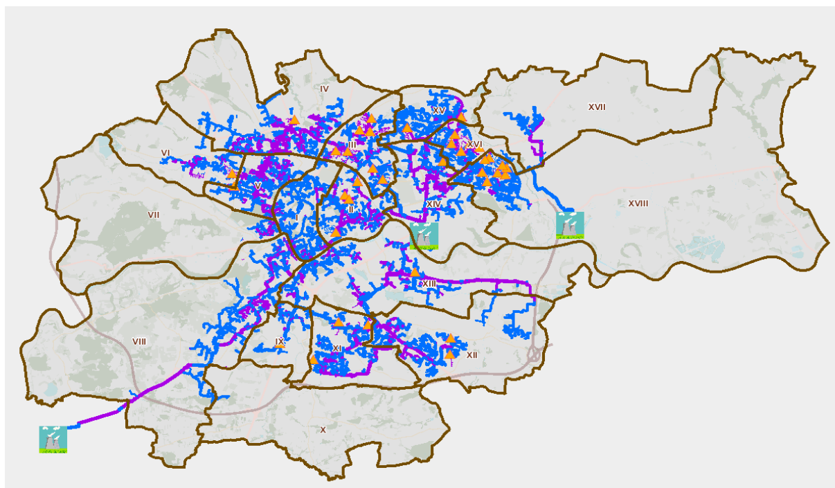
Rysunek 22 Mapa sieci ciepłowniczej na terenie miasta Kraków.
