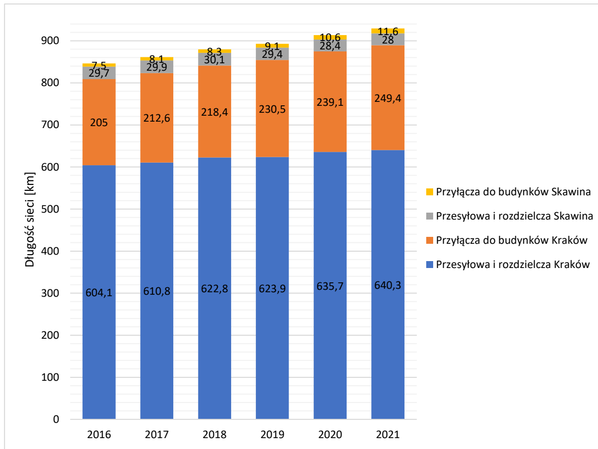
Rysunek 20 Długość sieci ciepłowniczej na terenie Krakowa oraz Skawiny.
