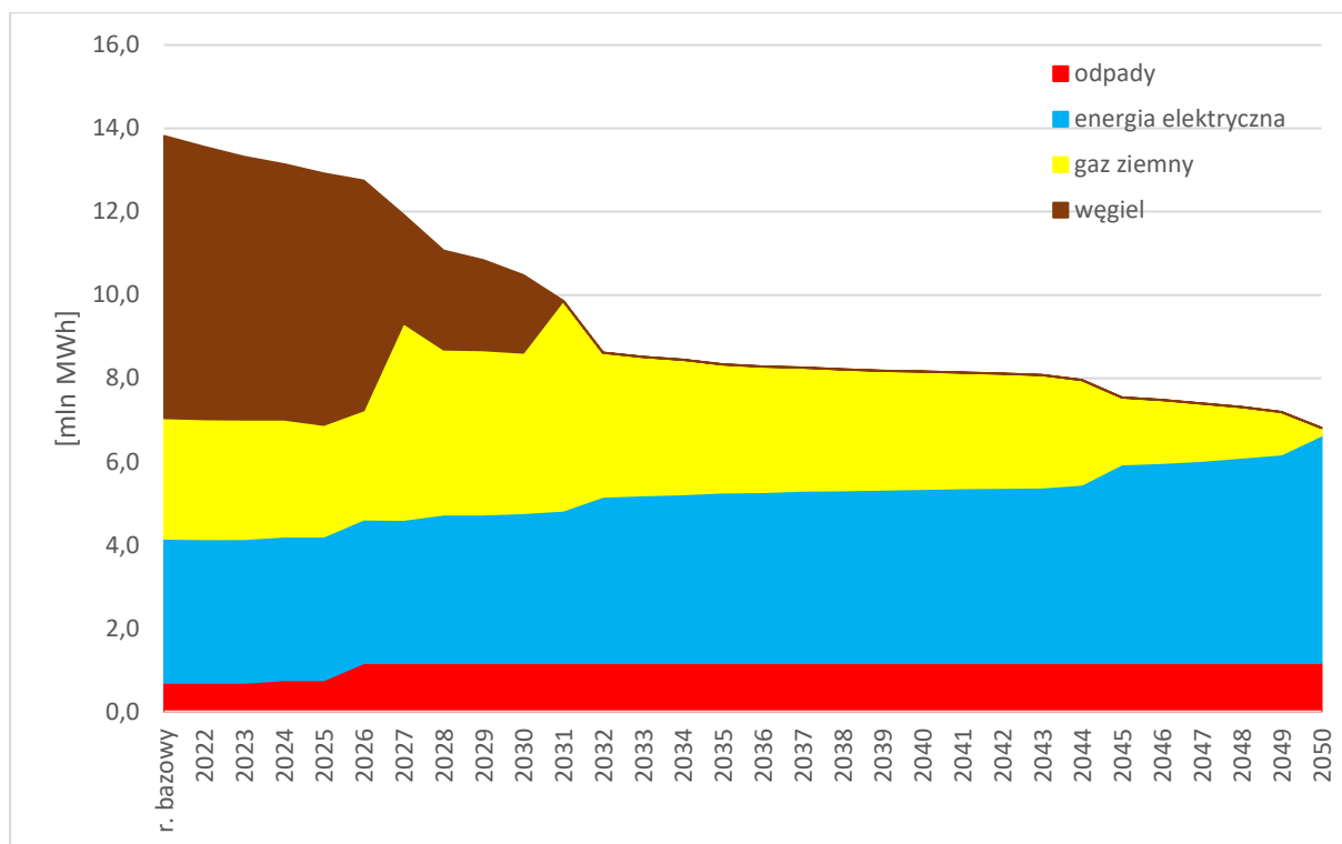
Rysunek 94 Zapotrzebowanie na nośniki energii dla całego miasta według Wariantu w latach 2021-2050.
