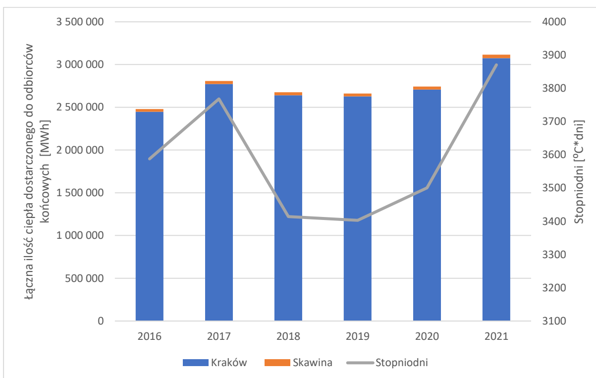
Rysunek 27 Łączna ilość ciepła dostarczonego do odbiorców końcowych na terenie gmin Kraków i Skawina w latach 2016-2021.
