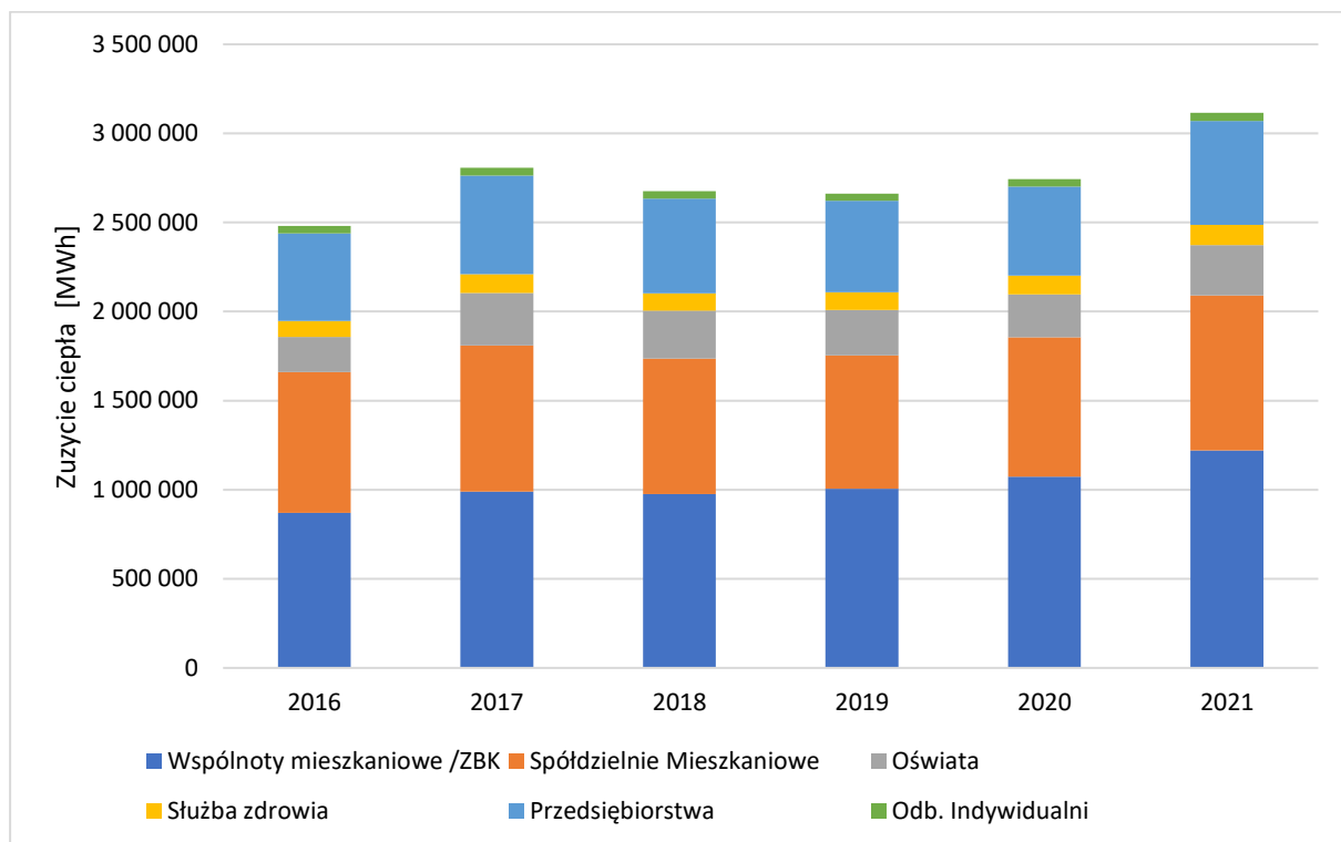
Rysunek 29 Zużycie ciepła przez poszczególne grupy odbiorców przyłączone do sieci ciepłowniczej MPEC S.A.
