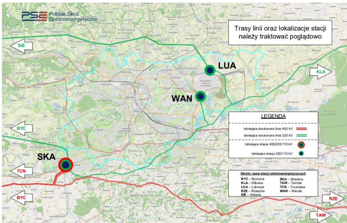
Rysunek 46 Schemat sieci przesyłowej na obszarze Gminy Miejskiej Kraków – stan istniejący. Źródło: PSE S.A.
