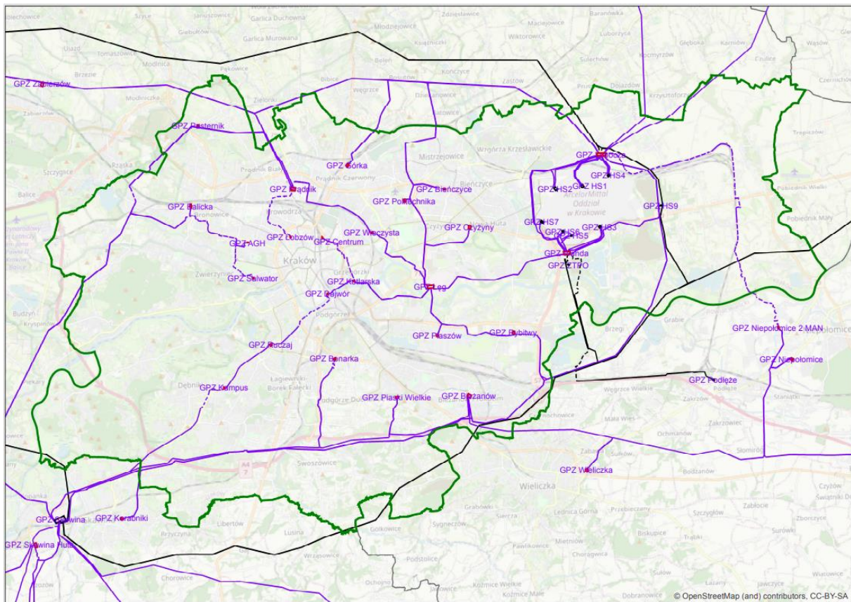
Rysunek 45 Plan istniejącej sieci przesyłowej najwyższych napięć wraz z zaznaczonymi Głównymi Punktami Zasilania.
