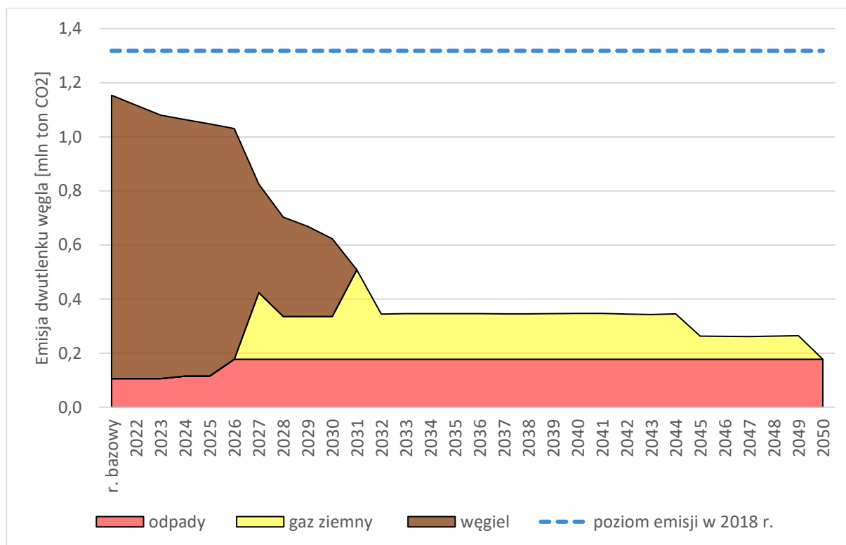
Rysunek 95 Poziomy emisji dwutlenku węgla (CO 2 ) z poszczególnych paliw używanych do produkcji ciepła dla miejskiej sieci ciepłowniczej według Wariantu w latach 2021-2050.
