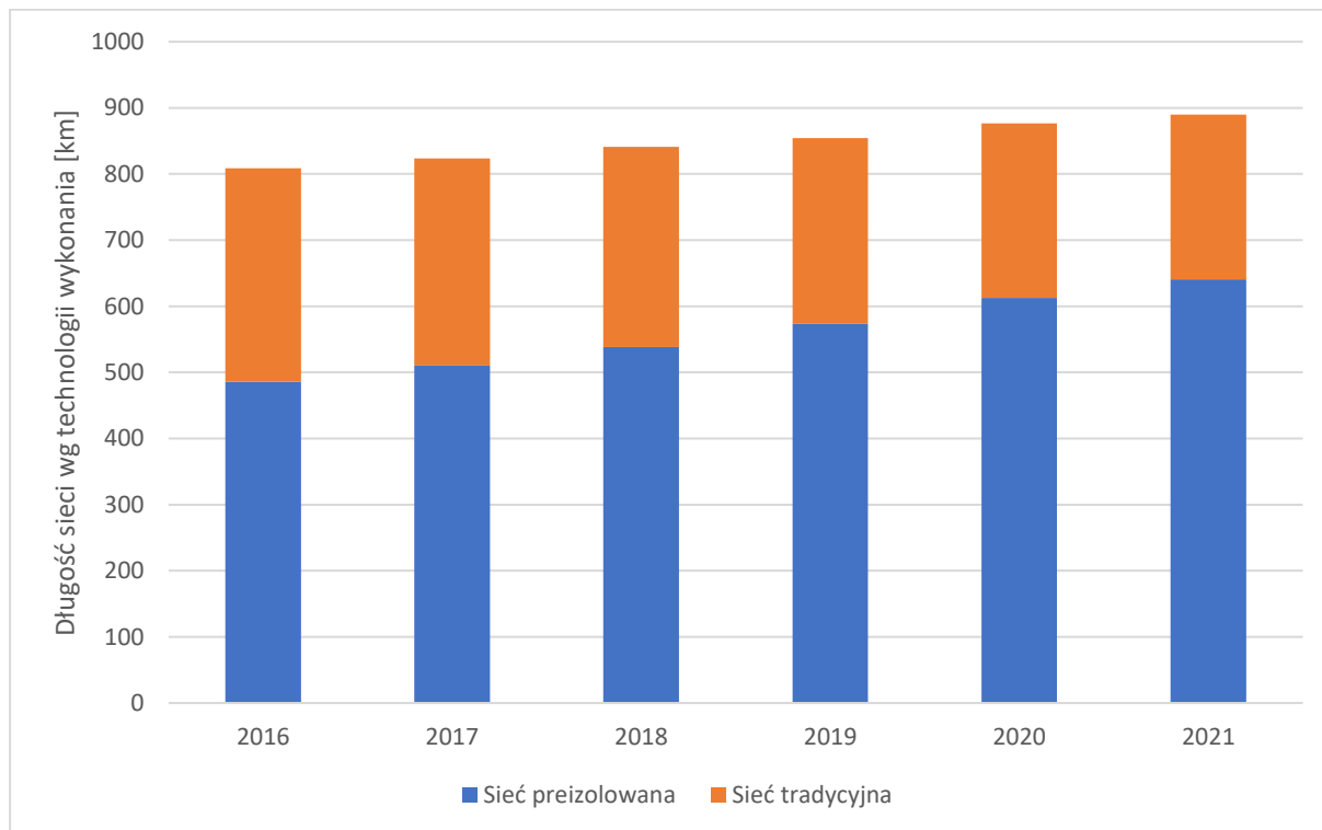
Rysunek 21 Sieć ciepłownicza na terenie Miasta Krakowa wg technologii wykonania.
