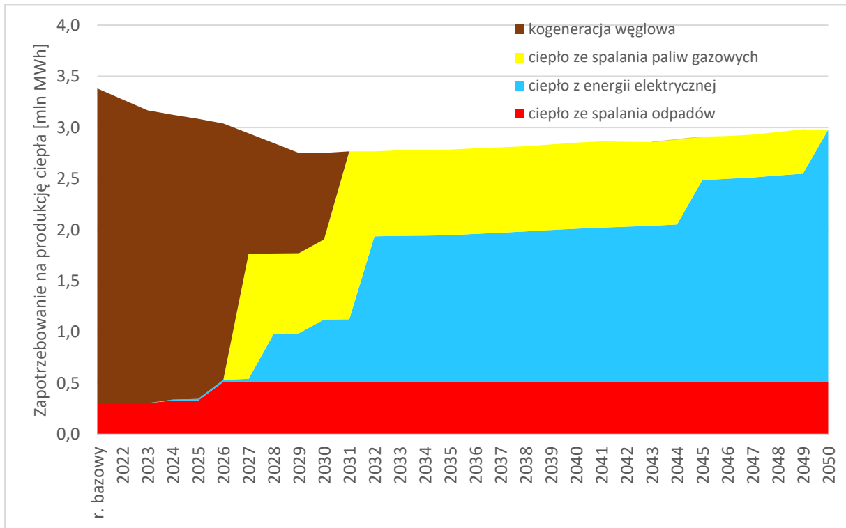
Rysunek 92 Zapotrzebowanie na produkcję ciepła dla msc w podziale na nośniki według Wariantu w latach 2021-2050.
