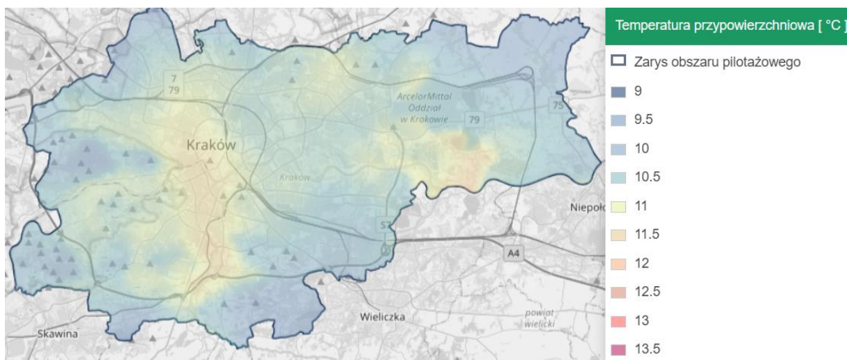
Rysunek 67 Temperatura podpowierzchniowa dla przedziału głębokości 0 - 100 m.
