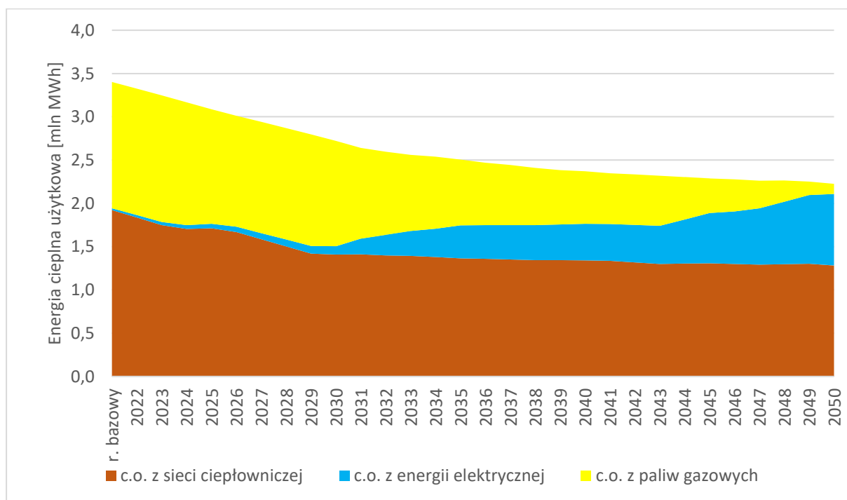
Rysunek 80 Prognoza zapotrzebowania na energię ciepłą użytkową na cele c.o. wśród zasobów budowlanych Krakowa w podziale na nośniki według Scenariusza 1 bazowego.
