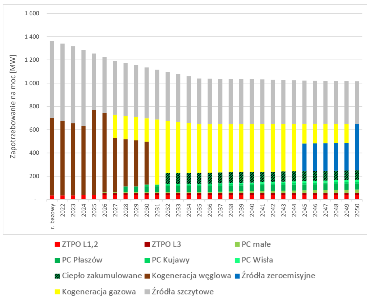
Rysunek 89 Zapotrzebowanie na moc w systemie ciepłowniczym w prognozowanym Wariancie w latach 2021-2050.
