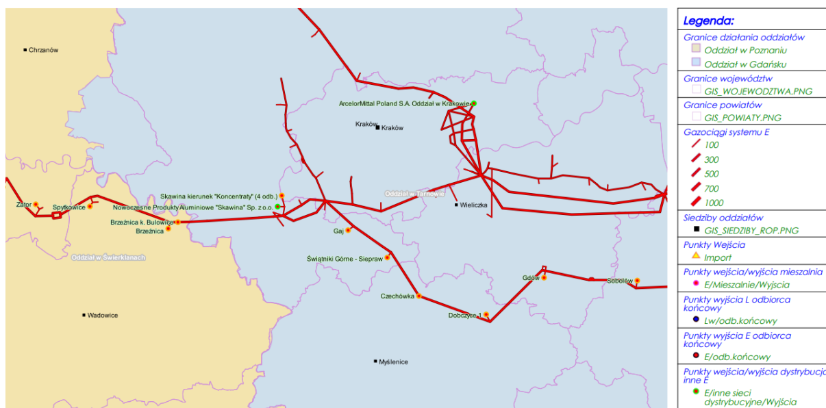
Rysunek 52 Mapa systemu przesyłowego GAZ-SYSTEM S.A. w Krakowie.
