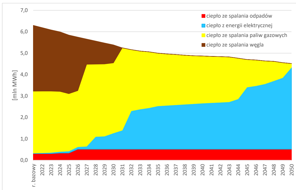
Rysunek 93 Zapotrzebowanie na produkcję ciepła dla całego miasta w podziale na nośniki według Wariantu w latach 2021-2050.
