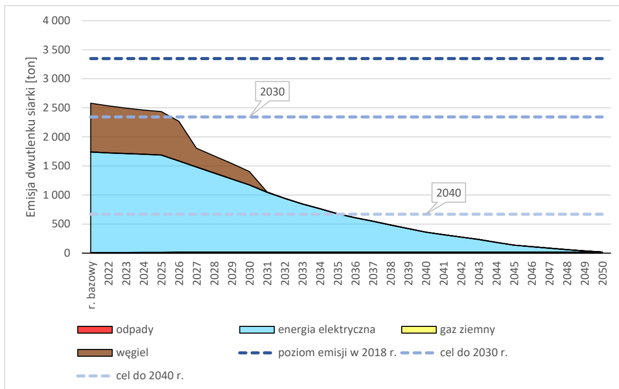
Rysunek 101 Emisja dwutlenku siarki (SO 2 ) wg Scenariusza 1 do 2050 r.
