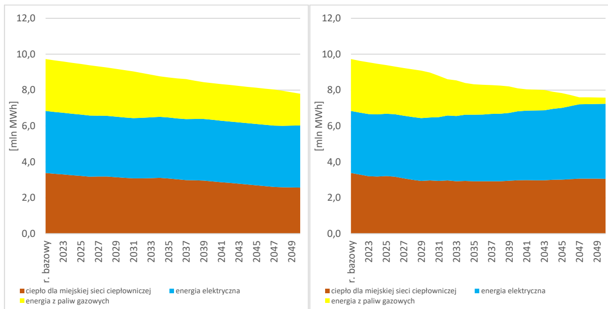
Rysunek 86 Progniza zapotrzebowania na nośniki energii w podziale na ciepło z miejskiej sieci ciepłowniczej, energię elektryczną i paliwa gazowe według Scenariusza 2 i 3.
