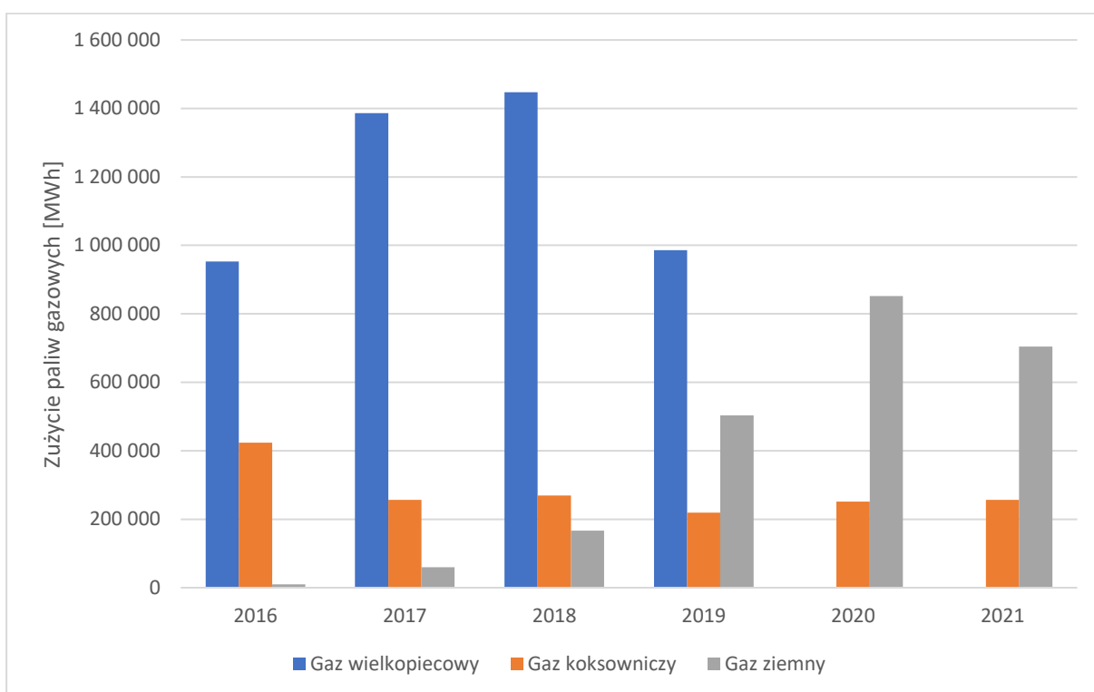
Rysunek 57 Zużycie paliw gazowych na potrzeby TAMEH POLSKA Zakład Wytwarzania Kraków na terenie Krakowa w latach 2016-2021.
