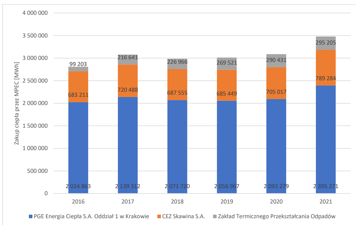
Rysunek 26 Zakup ciepła przez MPEC S.A. od poszczególnych wytwórców w latach 2016-2021 w celu zaspokojenia potrzeb odbiorców końcowych.
