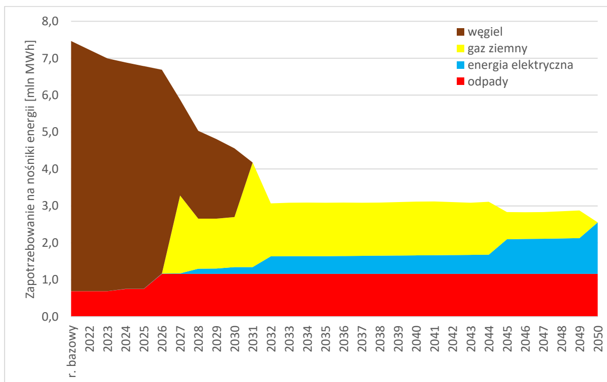
Rysunek 91 Zapotrzebowanie na nośniki energii dla miejskiej sieci ciepłowniczej według Wariantu w latach 2021-2050.
