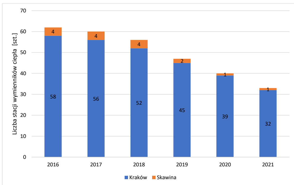
Rysunek 23 Liczba stacji wymienników ciepła na terenie Krakowa oraz Skawiny. Źródło: MPEC S.A. w Krakowie.
