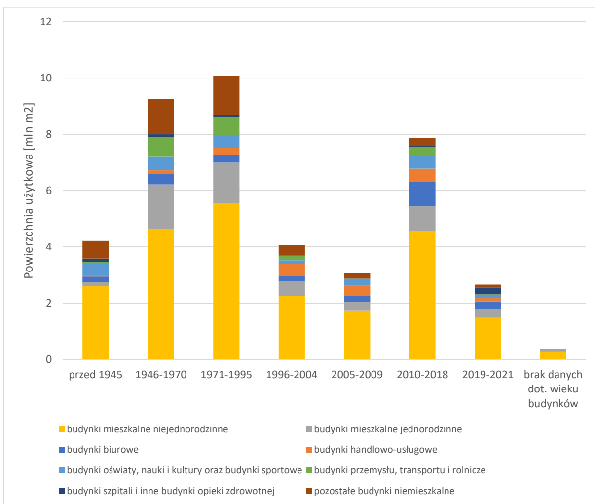
Rysunek 35 Struktura wiekowo-użytkowa zasobów budowlanych Krakowa według powierzchni ogrzewanej (stan na 12.2021 r.).
