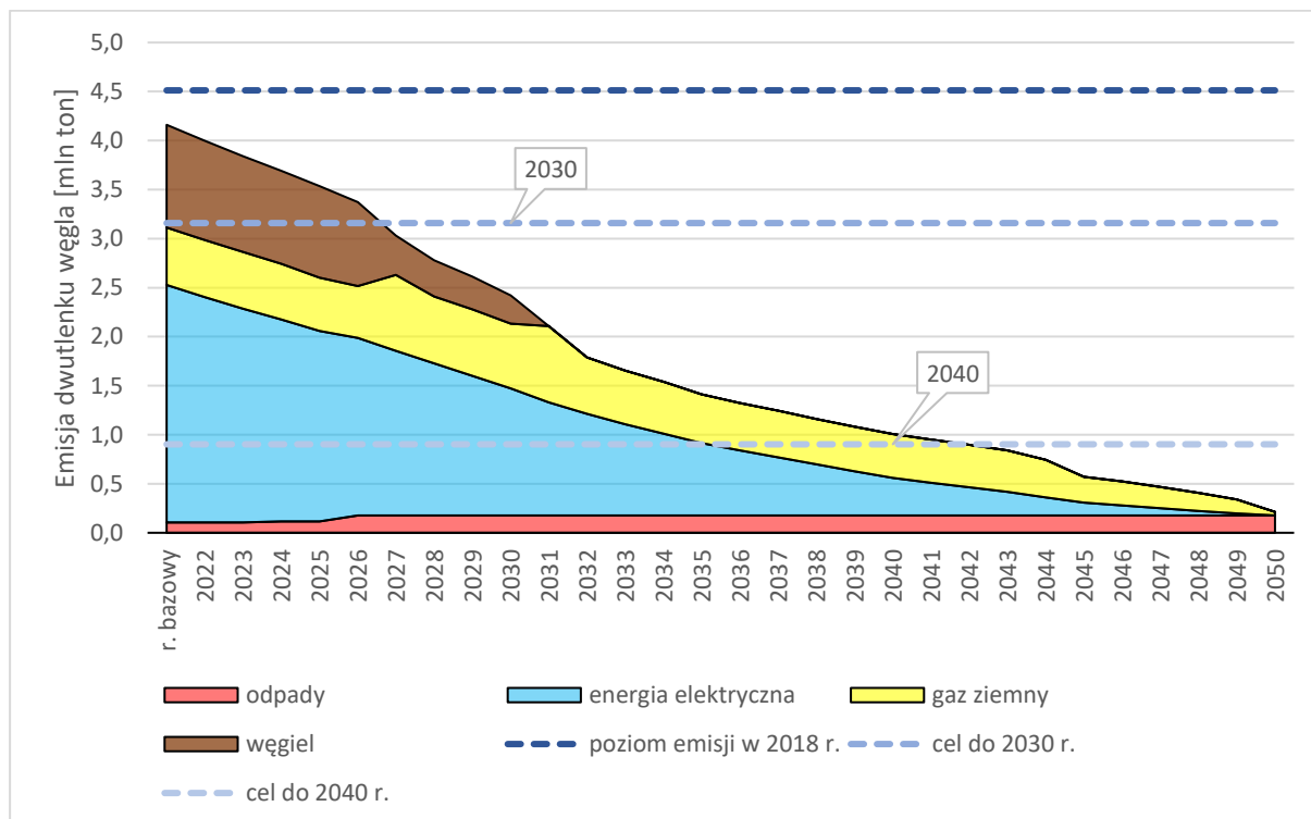
Rysunek 99 Emisja dwutlenku węgla (CO 2 ) wg Scenariusza 1 do 2050 r.
