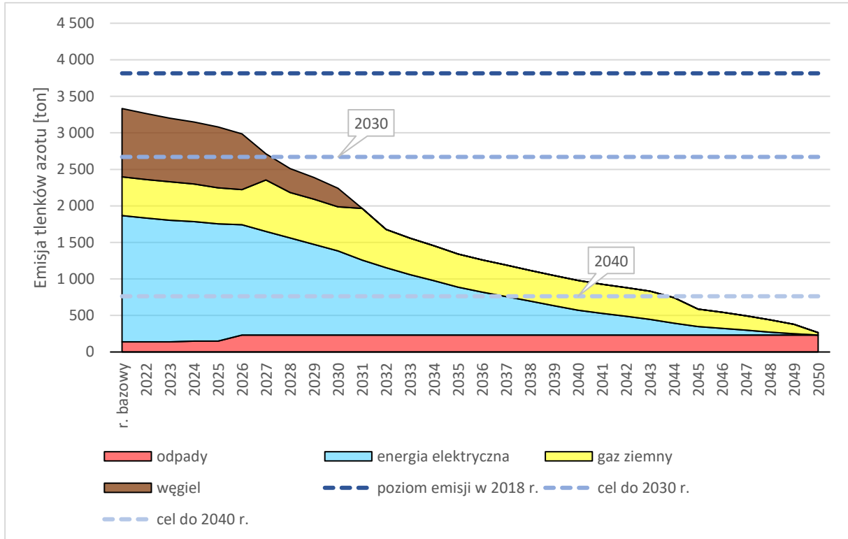
Rysunek 102 Emisja tlenków azotu (NOx) wg Scenariusza 1 do 2050 r.
