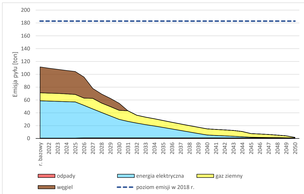
Rysunek 100 Emisja pyłu całkowitego (TSP) wg Scenariusza 1 do 2050 r.
