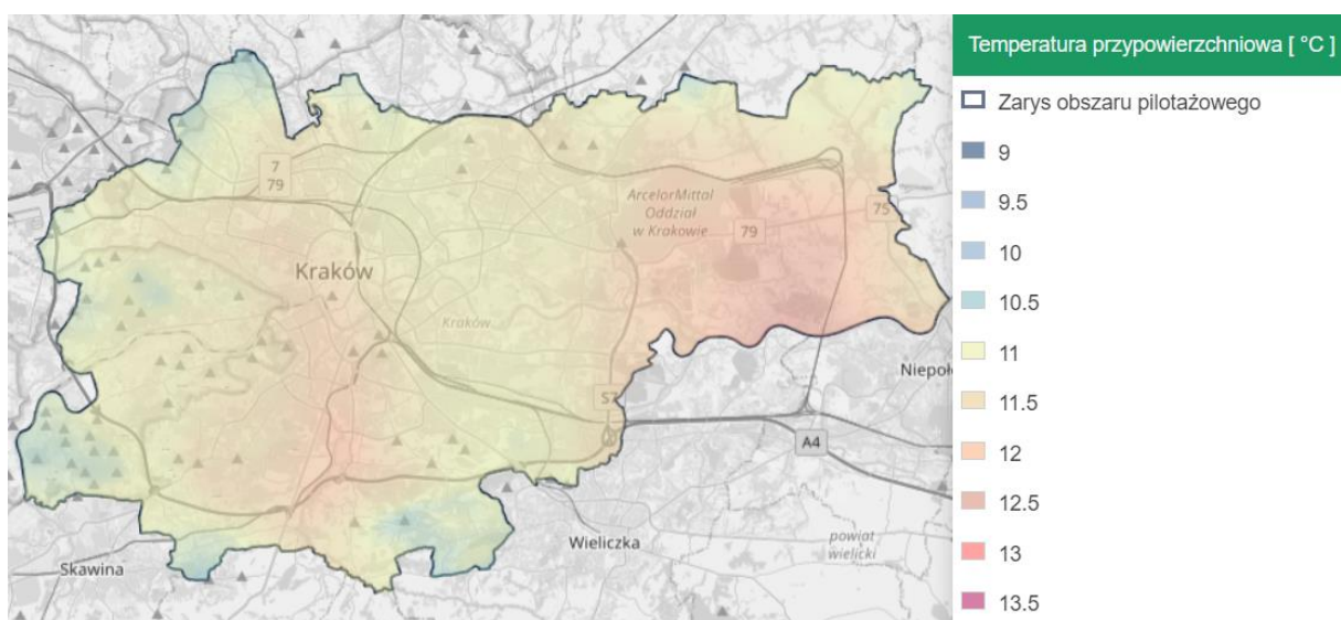
Rysunek 68 Temperatura podpowierzchniowa dla przedziału głębokości 0 - 150 m.
