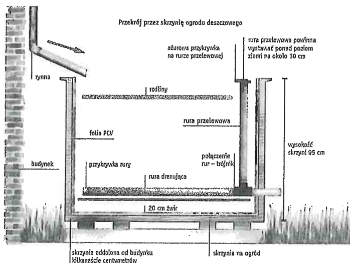
Rys.2. Przekrój przez przykładową skrzynię ogrodu deszczowego.
